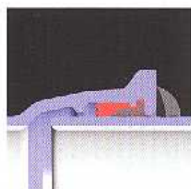
TYTON SIT PLUS® DIN 28603 DN 80-600
