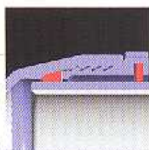
Csavaros, tokos csatlakozás kerék húzásbiztosítással DIN 28601 DN 80-400
