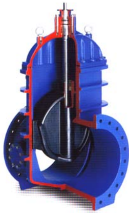
Tolózárok DN25 - 600
